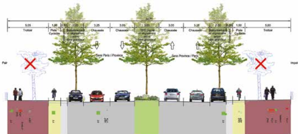
Coupe de principe sur Bourg-la-Reine, Bagneux, Arcueil et Cachan
